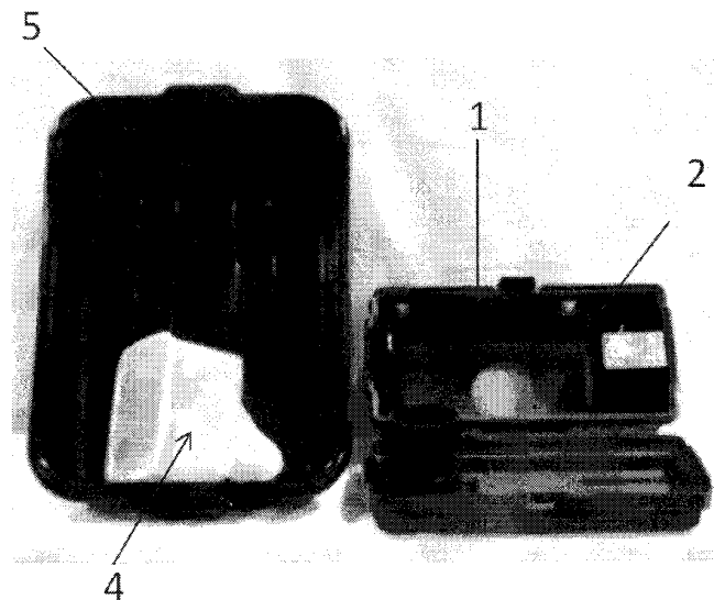
Figura 2: trappola tipo Gravid non assemblata.
