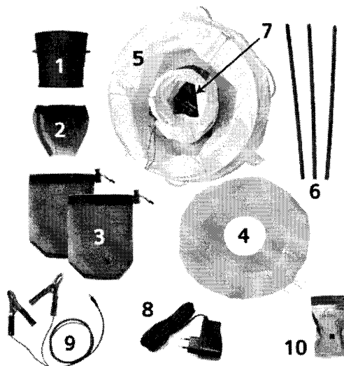
Figura 6: trappola BG-Sentinel non assemblata.
